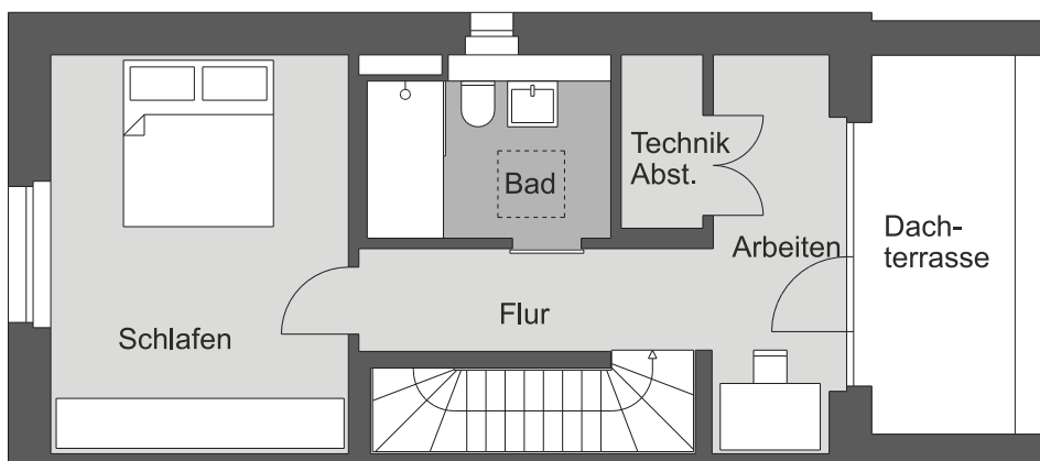
2. OG
