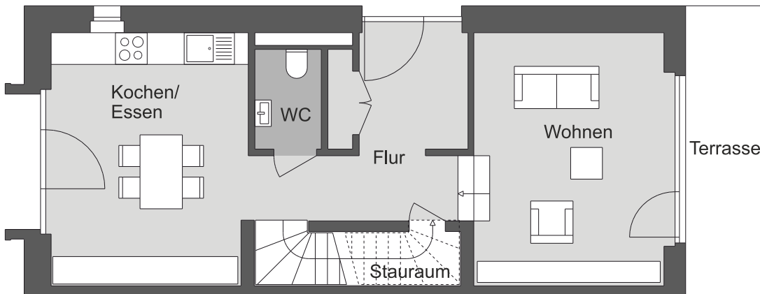
Erdgeschoss
