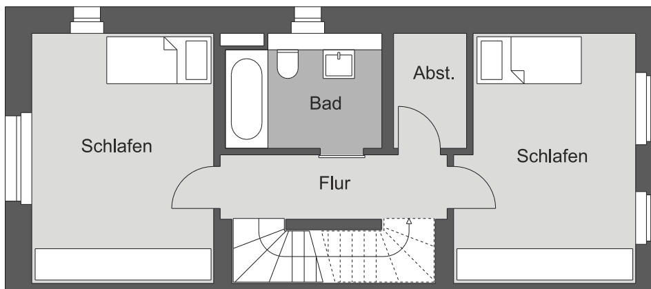
1. OG
